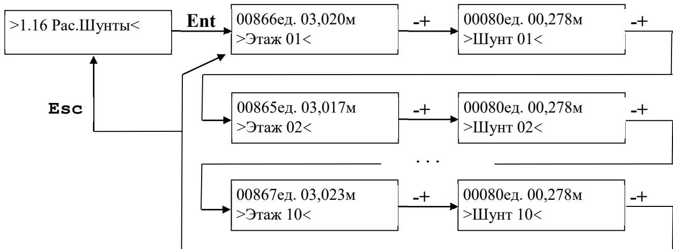
Рис. 18 Структура подменю >1.16 Рас.Шунты<
