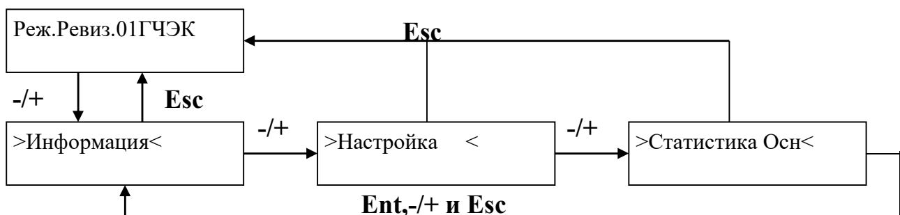
Рис. 3 Структура меню в режиме «РЕВИЗИЯ»
