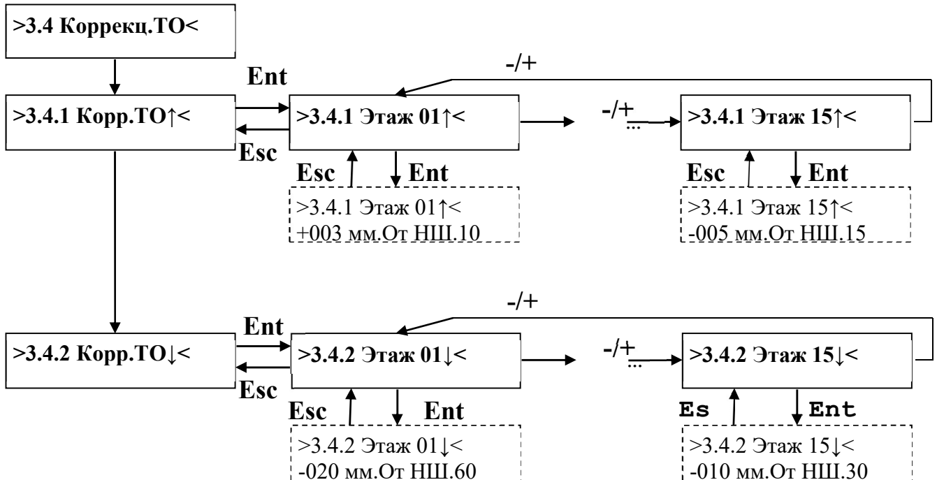
Рис. 28 Структура подменю >3.4 Коррекц.ТО<
