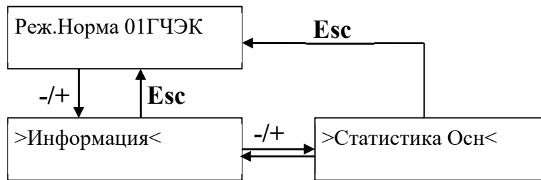
Рис. 2 Структура меню в режиме «НОРМА».
