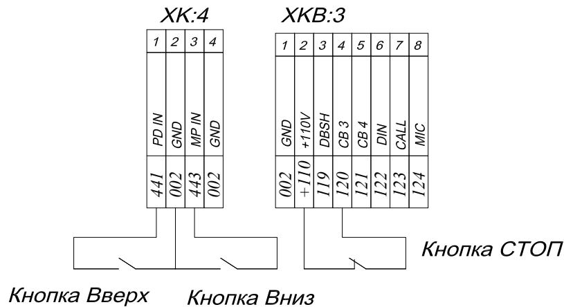
Рис. 29 Подключение поста ревизии.
