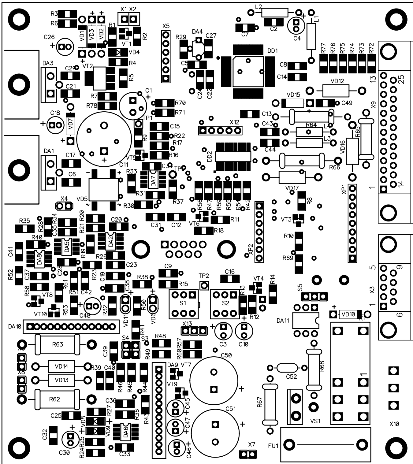
Блок лифтовой БЛ-50
